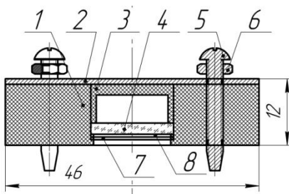
Рисунок 1 – Конструкция фантома
