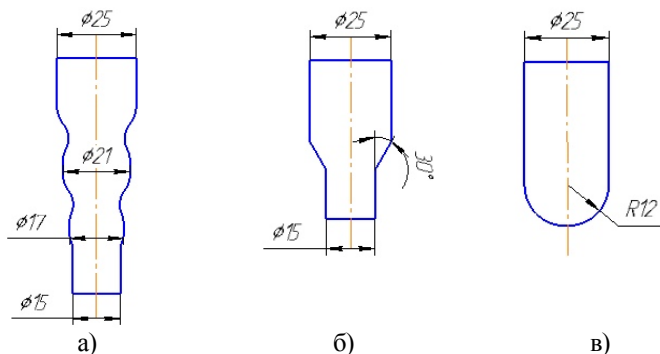
Рисунок 2 – Эскиз деформирующих инструментов
