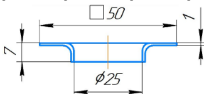
Рисунок 1 – Геометрические характеристики детали
