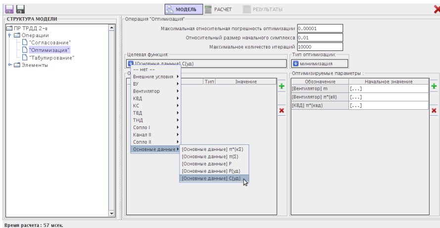
Рисунок 10 — Панель редактирования свойств операции «Оптимизация»
