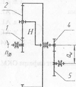
Рисунок Б2 - Схема редуктора
