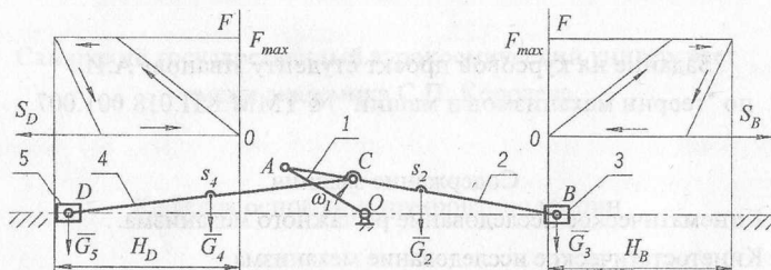
Рисунок Б1 - Схема компрессора
