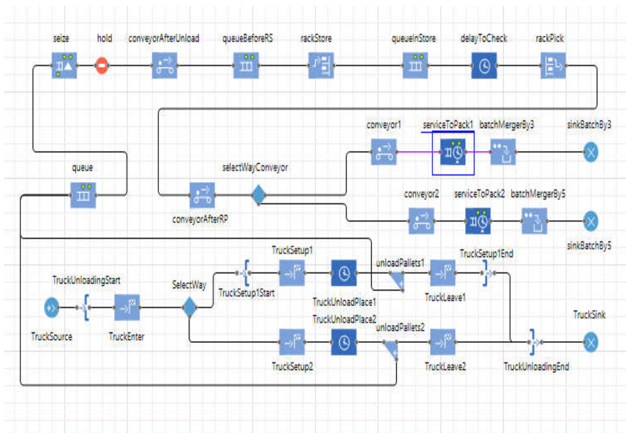
Рис. 2. Модель работы распределительного центра в системе AnyLogic
