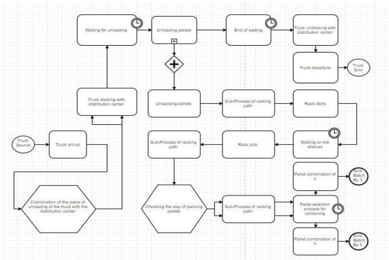
Рис. 1. Диаграмма работы распределительного центра
