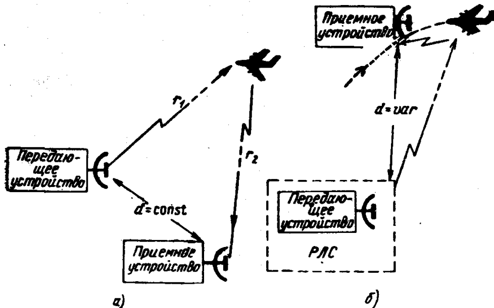
Рис.1.4.Активная радиолокационная система
