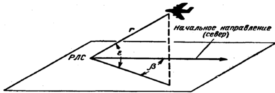
Рис.1.1 Сферические координаты цели
