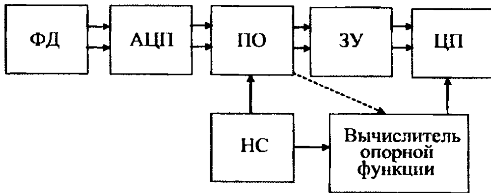
Рис. Цифровая система обработки
