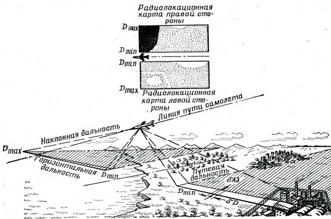
Рис.Обзор земной поверхности РЛС бокового обзора
