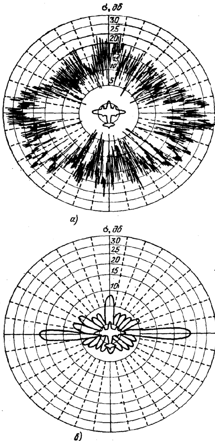
Рис.1.5. Диаграмма переизлучения самолета при \lambda = 10 см (а) и \lambda = 3 м (б)
