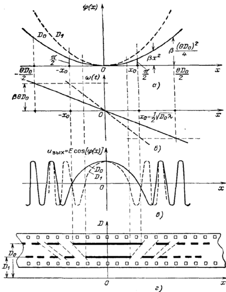
Рис. Характер изменения сигнала, отраженного от цели в РЛС с синтезированным раскрытием в зависимости от значений переменной X
