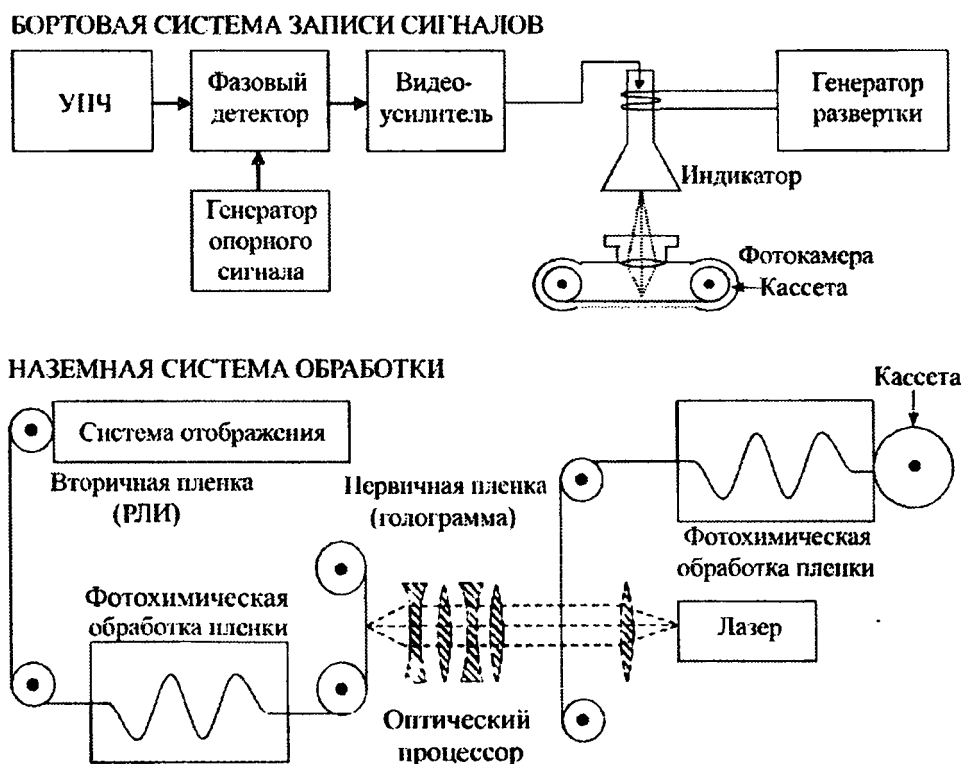
Рис. Структурная схема бортовой и наземной частей оптической системы записи и обработки сигналов в РСА
