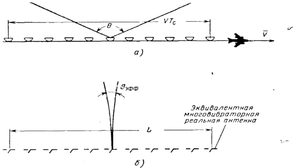
Рис. Принцип формирования искусственного ( синтезированного ) раскрытия .
