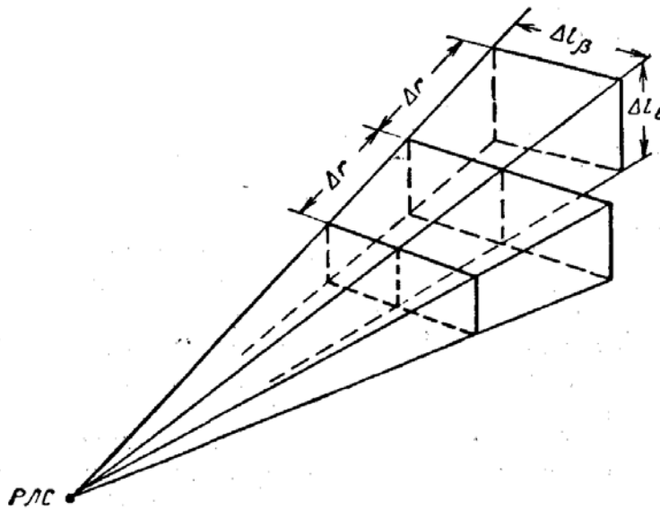
Рис.1.2.Разрешаемый объем радиолокатора
