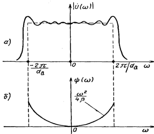
Рис. Амплитудный (а) и фазовый (б) спектры сигнала
