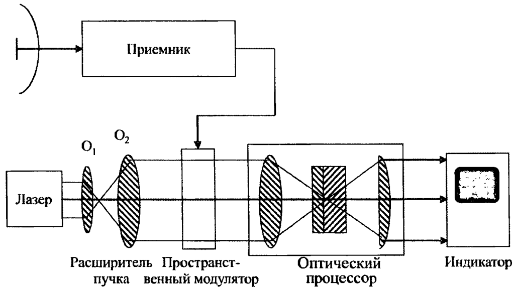
Рис. Схема оптической обработки сигналов РСА
