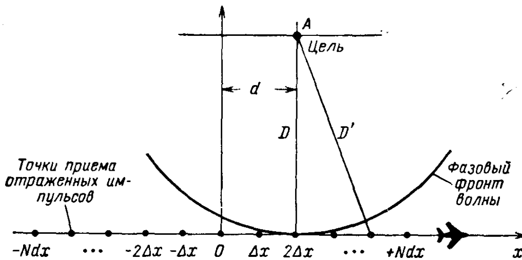
Рис. Формирование синтезированного раскрыва при импульсном характере сигналов РЛС
