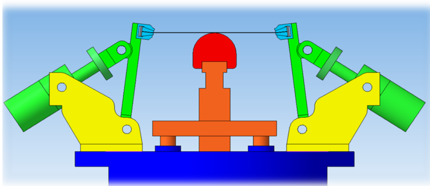
Рис. 6.2. Схема лабораторного обтяжного пресса (начальное положение рабочих органов)
