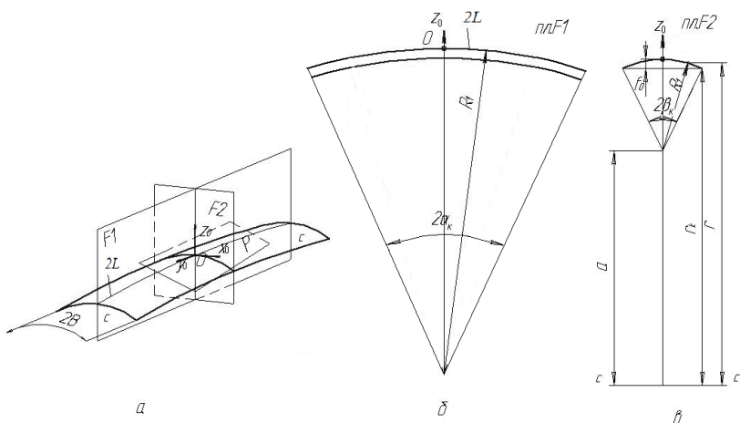
Рис. 2.4. «Пологая» оболочка двояковыпуклой формы, характеризующаяся следующими значениями L/B \geq 10 и 2\alpha_{\kappa} \leq 60^\circ : а – поверхность оболочки двойной кривизны; б – формообразующий продольный контур; в – центральный поперечный контур
