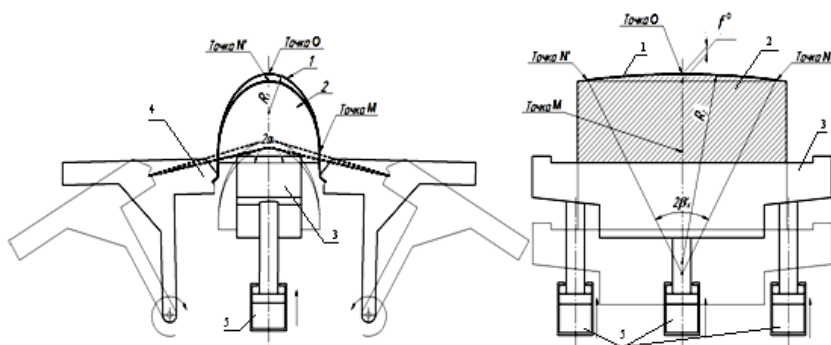
Рис. 5.3. Схема разгрузки и изгибания на прессе FEKD 550-1100 оболочки с полным охватом обтяжного пуансона:
