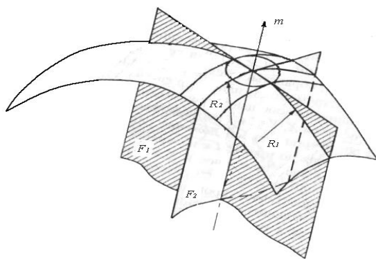
Рис. 2.2. Метод определения положения нормали для обработки строки поверхности обтяжного пуансона с помощью ортогональных плоскостей F_1 и F_2
