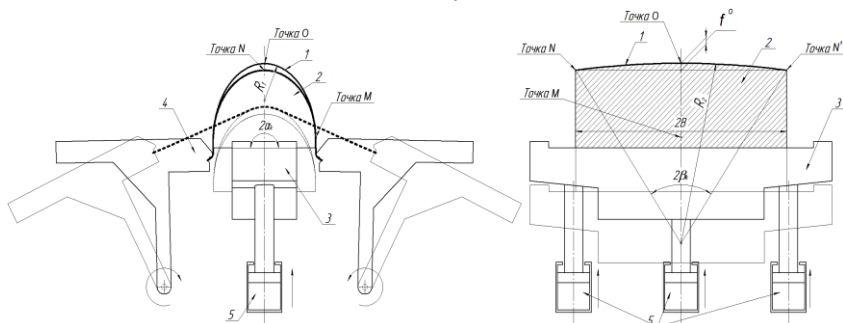
Рис. 5.1.Схема стадии предварительной обтяжки на прессе FEKD 550-1100: 1 – листовая заготовка; 2 – обтяжной пуансон; 3 – рабочий стол пресса; 4 – балансиры; 5 – силовые гидроцилиндры стола пресса
