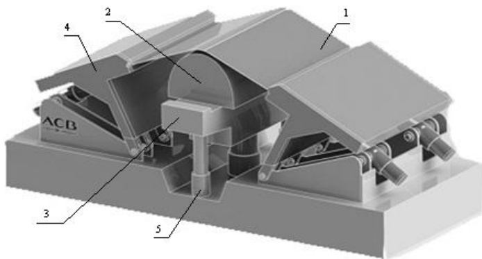
Рис. 5.4. Обтяжной пресс поперечного действия типа FEKD
