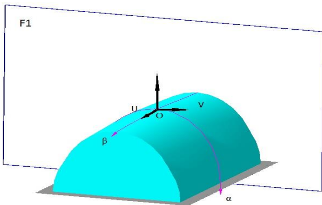
Рис. 2.6. Положение прямоугольного контура основания обтяжного пуансона относительно поверхности обшивки, обеспечивающее постоянное положение формообразующего контура в вертикальной плоскости симметрии F_1
