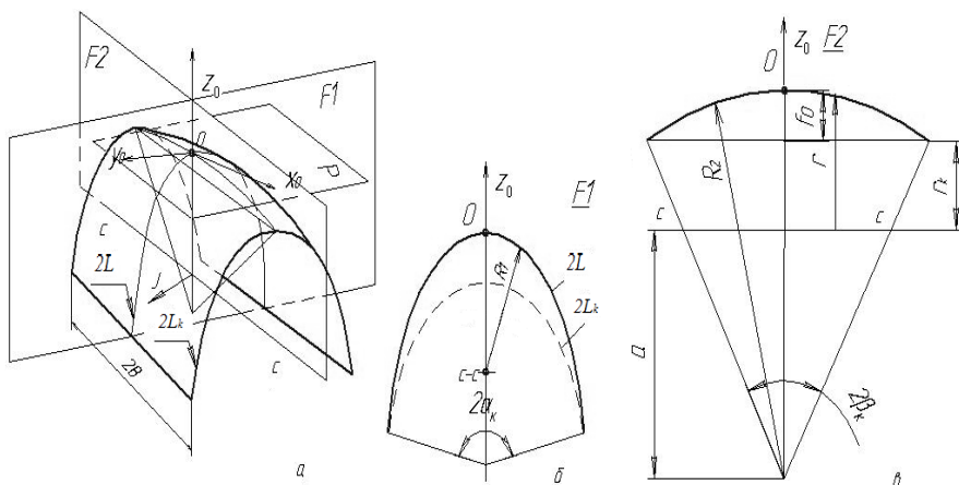
Рис. 2.5. «Крутая» оболочка двояковыпуклой формы, характеризующаяся следующими значениями L/B \leq 1,0 и 2\alpha_{\kappa} > 120^\circ : а – поверхность оболочки двойной кривизны; б – формообразующий продольный контур; в – центральный поперечный контур
