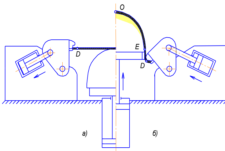
Рис.б.1. Кинематика прессы типа FEKD и схема обтяжки: а – начальное положение; б – конечное положение
