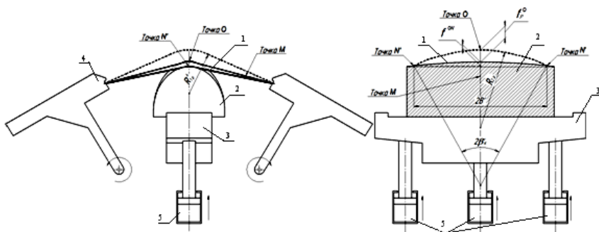
Рис. 5.2. Схема стадии повторной обтяжки на прессе FEKD 550-1100: 1 – листовая заготовка; 2 – обтяжной пуансон; 3 – рабочий стол пресса; 4 – балансир; 5 – силовые гидроцилиндры стола пресса
