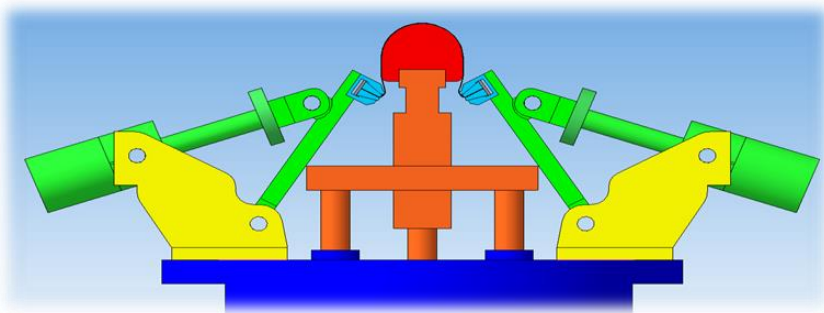
Рис. 6.3. Схема лабораторного обтяжного пресса (конечное положение рабочих органов)
