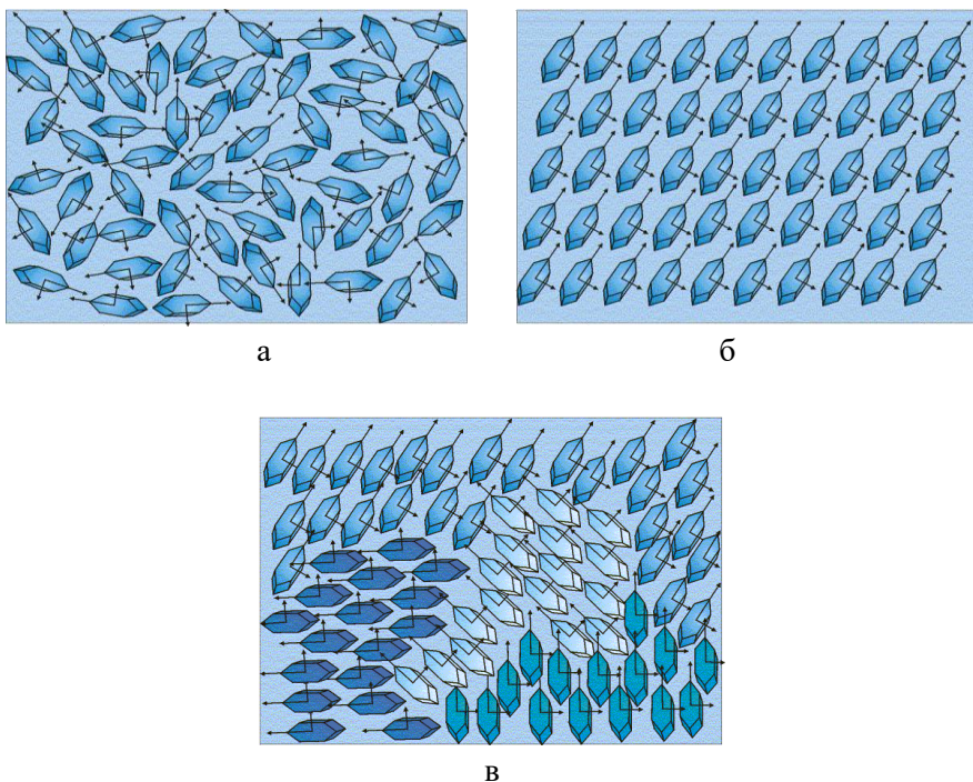
Рис. 1.2. Текстуры прокатки:
