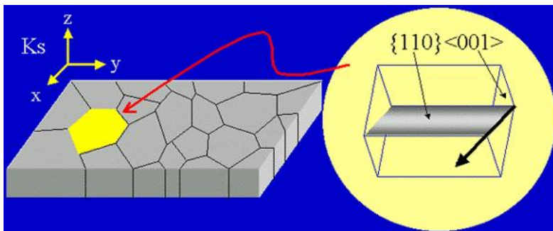
Рис. 1.1. Пример индексации кристаллографических плоскостей и направлений листового проката
