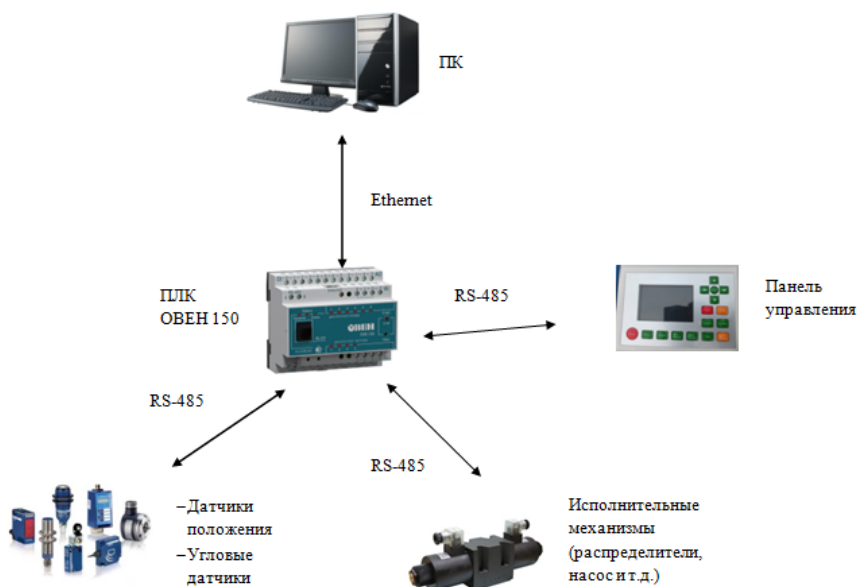
Рис.6.5. Структура системы управления
