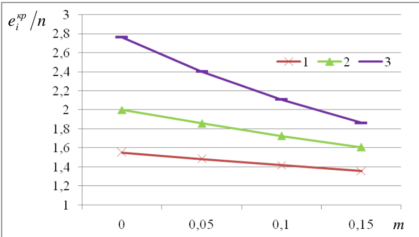
1 – \Delta_1 = 0,248, \Delta_2 = 0,333, \Delta_3 = 0,250 ( \{011\} < 211 > ); 2 – \Delta_1 = \Delta_2 = \Delta_3 = 0,2 (изотропная среда); 3 – \Delta_1 = 0,240, \Delta_2 = 0,103, \Delta_3 = 0,186 ( \{124\} < 211 > )
