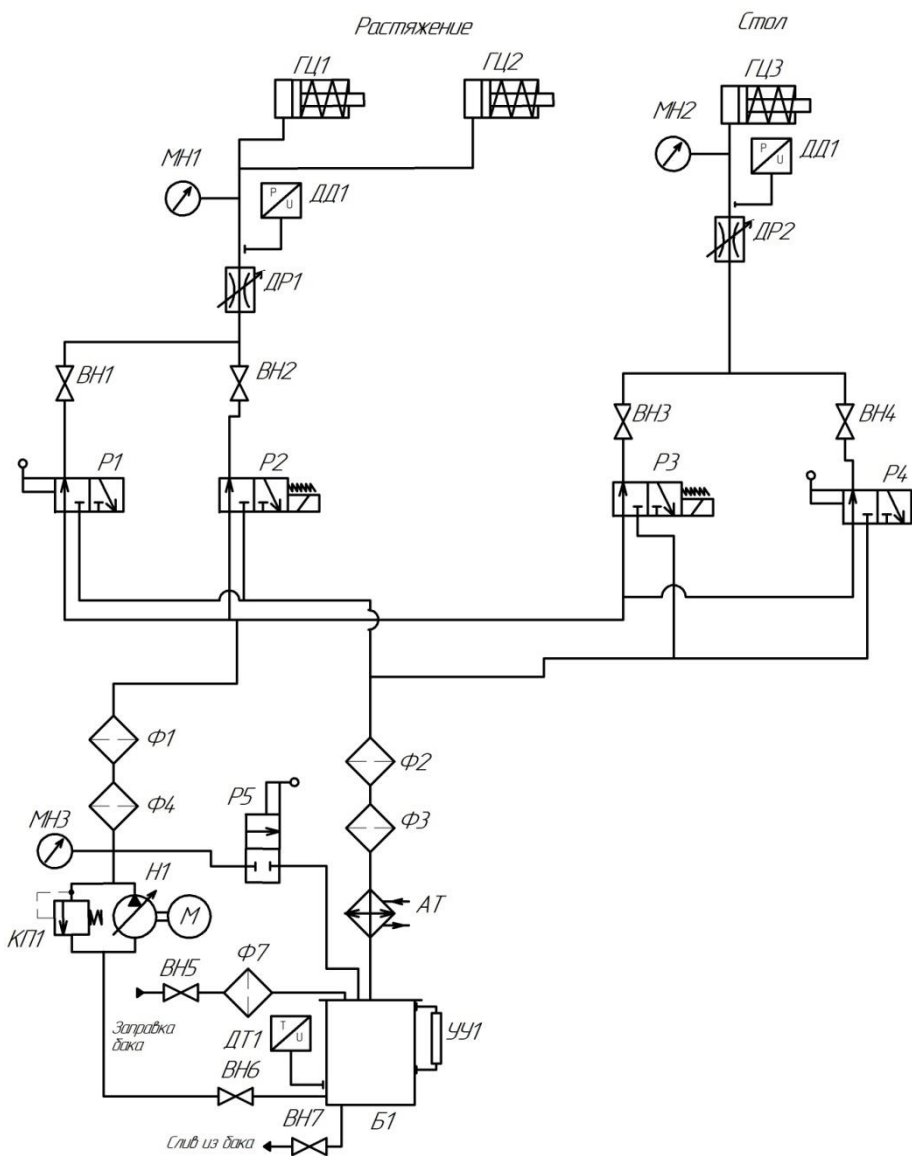
Рис. 6.4. Гидравлическая система лабораторного обтяжного пресса
