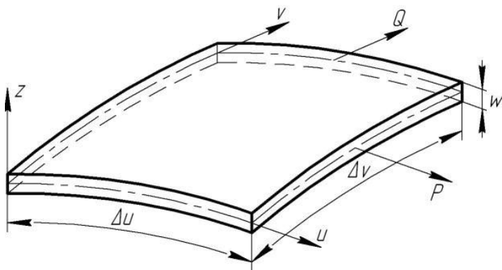
Рис. 4.1. Элемент анизотропной заготовки, находящейся в двухосном напряженном состоянии
