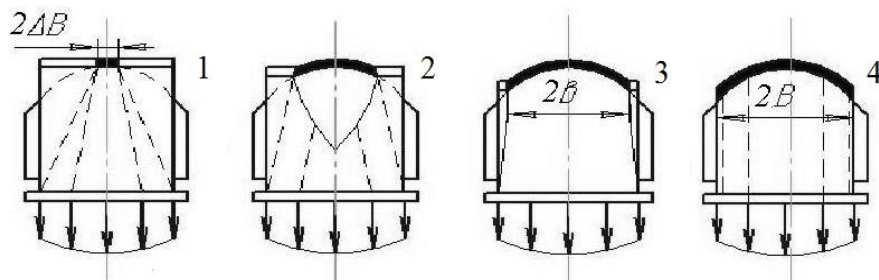
Рис. 3.1. Предварительная обтяжка оболочки двояковыпуклой формы после полного оборачивания обтяжного пуансона листовой заготовкой на угол \alpha_k
