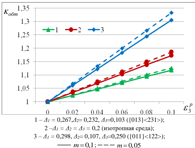
Рис. 4.3. Взаимосвязь между напряженным состоянием m , деформацией утонения \varepsilon_3^p , геометрическим коэффициентом обтяжки K_{обт} и текстурными параметрами \Delta_i
