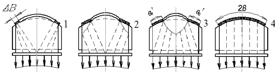
Рис. 3.2. Повторная обтяжка оболочки двояковыпуклой формы после ее разгиба на угол \alpha_p
