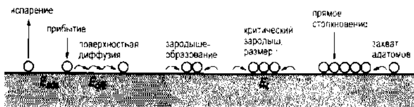
Рис. 20. Схематическая диаграмма, иллюстрирующая атомные процессы, задействованные в зарождении и росте островков на поверхности
