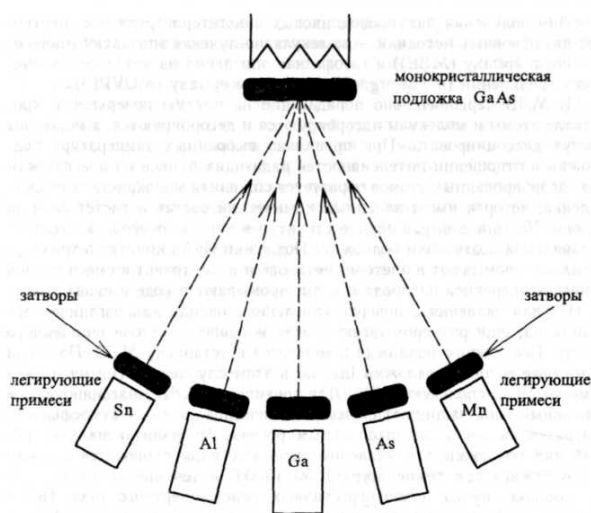
Рис. 27. Схема установки для молекулярно-лучевой эпитаксии:
