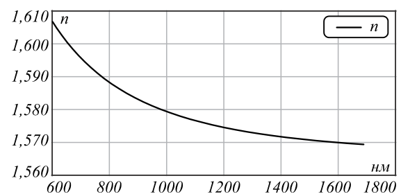
Рис. 1. Показатель преломления резиста ФП-3535
