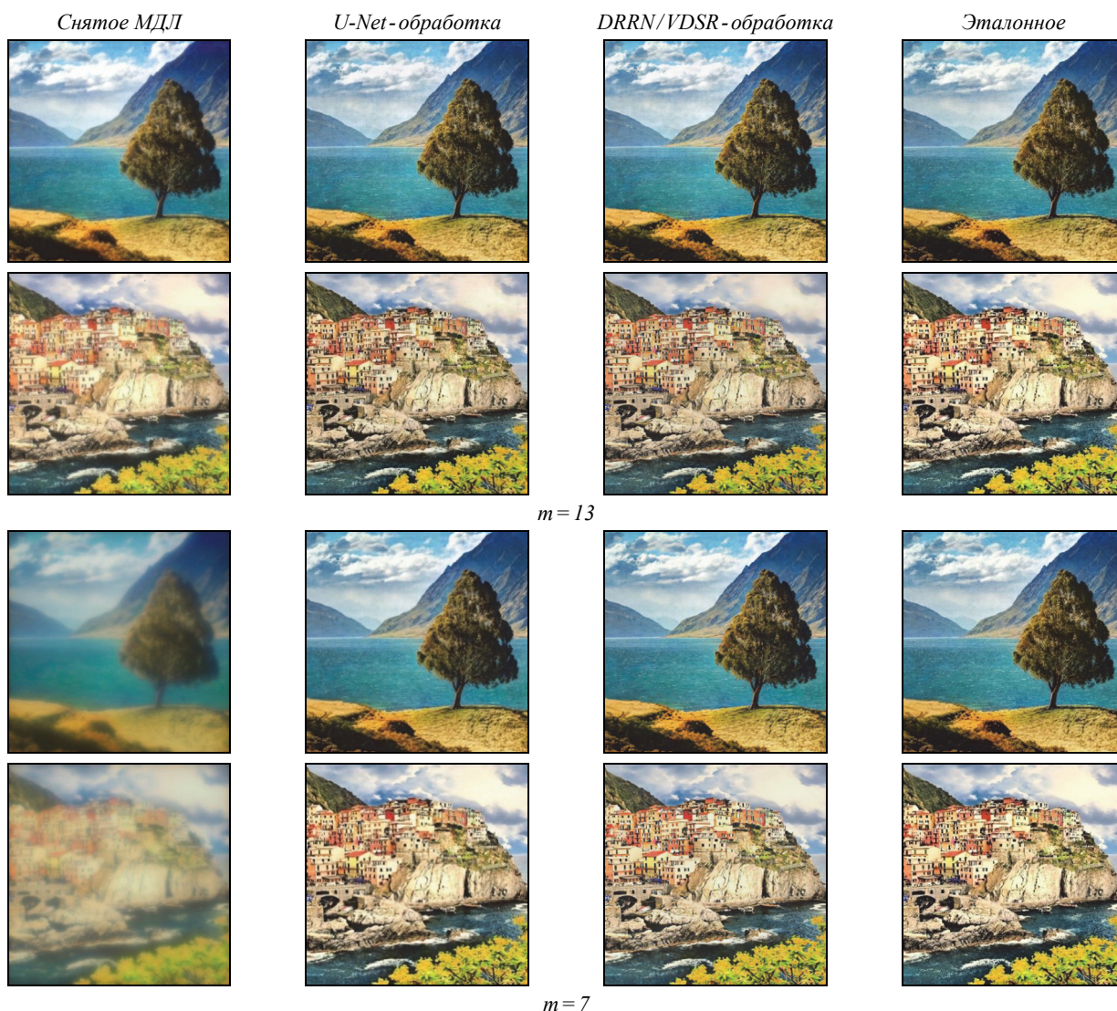
Рис. 10. Примеры изображений из тестовой выборки для m = 13 и m = 7
