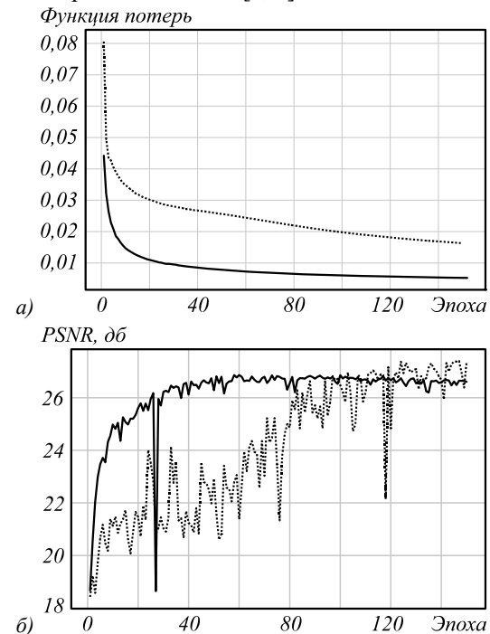
Рис. 7. Графики зависимости функции потерь (а) и PSNR (б) на валидационной выборке
