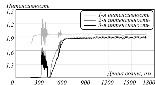
Рис. 2. Спектральный коэффициент пропускания резиста ФП-3535
