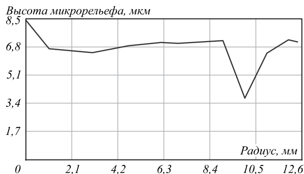
Рис. 4. Зависимость высоты микрорельефа от радиуса записи
