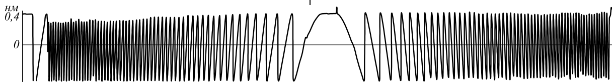
Рис. 3. Профилограмма дифракционной линзы с высотой микрорельефа 7,5 мкм
