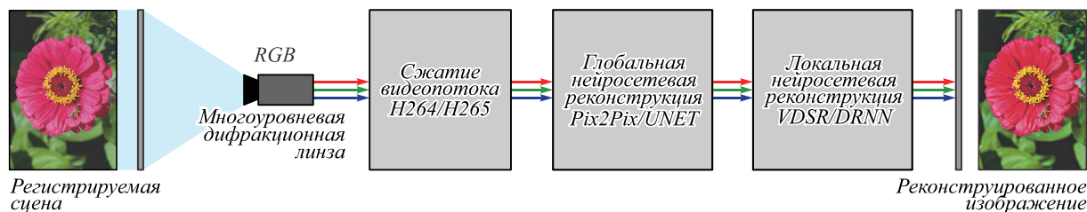
Рис. 6. Нейросетевая реконструкция видеопотока
